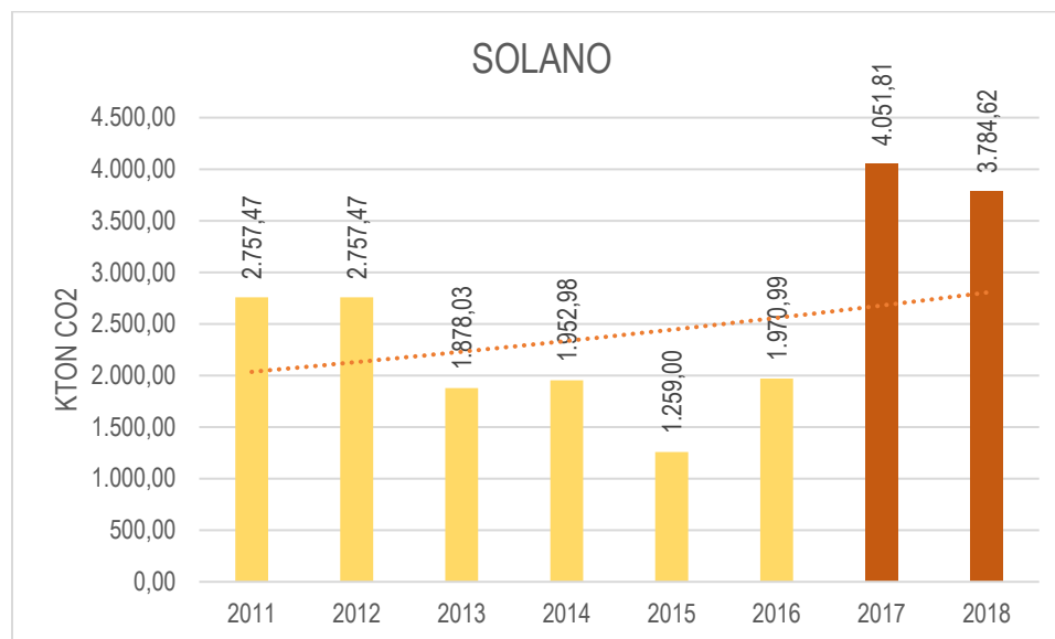
FIGURA 21. EMISIONES DE CO2 POR DEFORESTACIÓN, EN EL MUNICIPIO DE SOLANO DURANTE EL PERIODO 2011-2018
