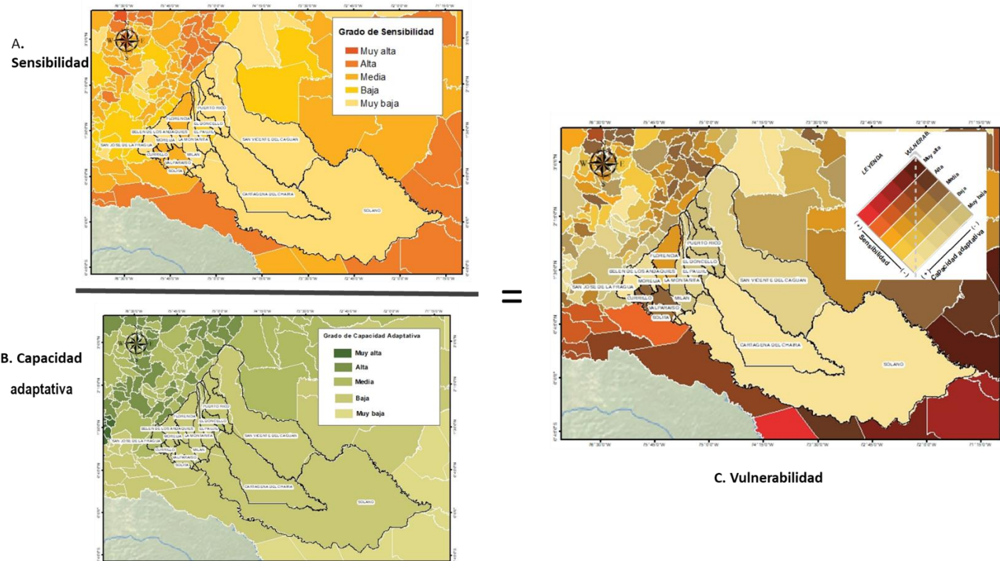
FIGURA 27. MAPA DE VULNERABILIDAD AL CAMBIO CLIMÁTICO PARA EL DEPARTAMENTO DEL CAQUETÁ TCNCC. A. SENSIBILIDAD. B. CAPACIDAD ADAPTATIVA, C. VULNERABILIDAD
