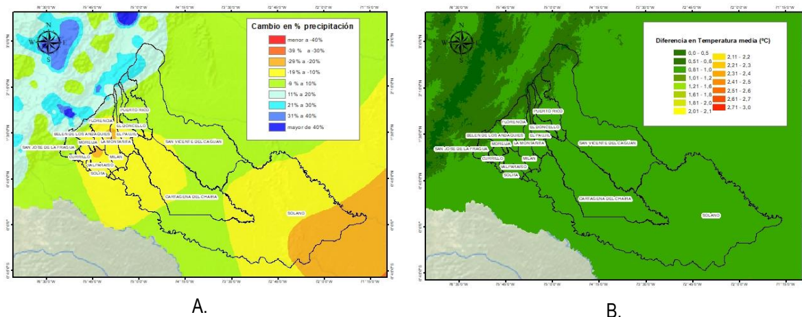
FIGURA 24. A) ESCENARIO DE CAMBIO 2011-2040 EN PORCENTAJE DE PRECIPITACIÓN (%) PARA EL DEPARTAMENTO DE CAQUETÁ. B) ESCENARIO DE CAMBIO 2011-2040 DE DIFERENCIA DE TEMPERATURA PARA EL DEPARTAMENTO DE CAQUETÁ
