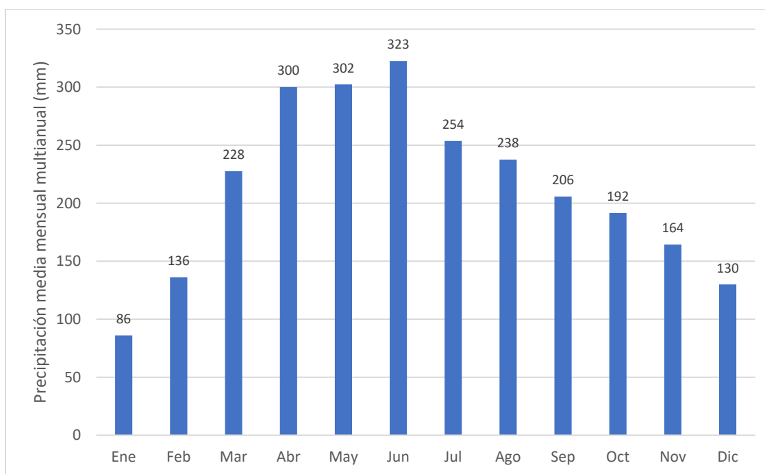
FIGURA 18. VARIACIÓN MENSUAL MULTIANUAL DE LA PRECIPITACIÓN PARA LA ESTACIÓN TRES ESQUINAS
