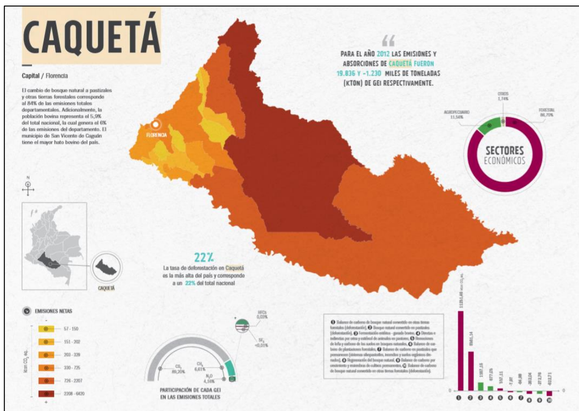
FIGURA 20. EMISIONES Y ABSORCIONES DE GEI DEL DEPARTAMENTO DE CAQUETÁ
