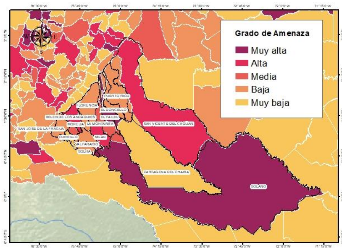
FIGURA 26. MAPA DE AMENAZA POR CAMBIO CLIMÁTICO PARA EL DEPARTAMENTO DE CAQUETÁ. TCNCC
