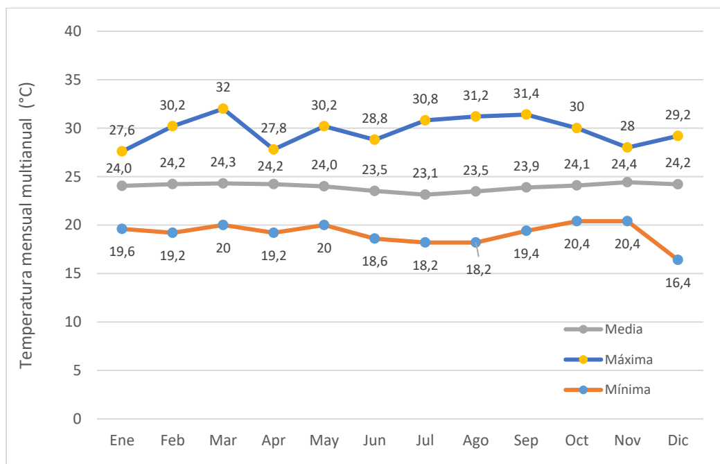
FIGURA 16. VARIACIÓN MENSUAL MULTIANUAL DE LA TEMPERATURA PARA LA ESTACIÓN PTO LEGUIZAMO
