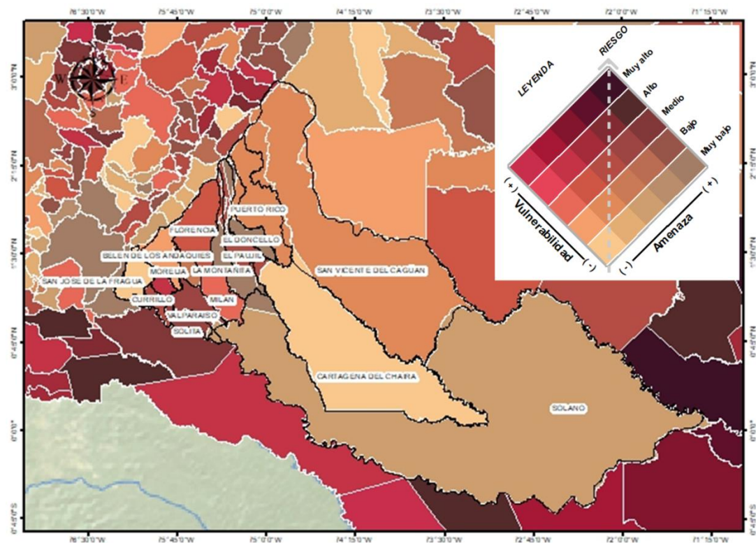
FIGURA 28. MAPA DE RIESGO AL CAMBIO CLIMÁTICO PARA EL DEPARTAMENTO DEL CAQUETÁ TCNCC
